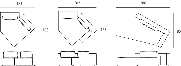
9YA602 Elemento angolare Corner element L184 P185 H66 9YA604 Elemento angolare Corner element L202 P185 H66 9YA605 Elemento angolare Corner element L286 P185 H66
