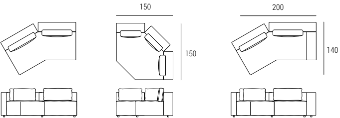
9YA601 Elemento angolare Corner element L200 P140 H66 9YA603 Elemento angolare Corner element L150 P150 H66 9YA607 Elemento angolare Corner element L225 P140 H66
